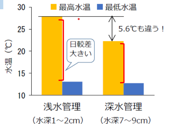
図 水田の水深と水温の関係
